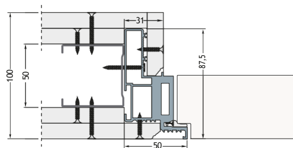
Tokszerkezet két gipszkarton lappal (50 mm-es bordához): Kész fal vastagsága 100 mm
