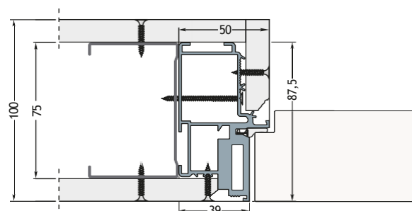
Tokszerkezet egy gipszkarton lappal: Kész fal vastagsága 100 mm
