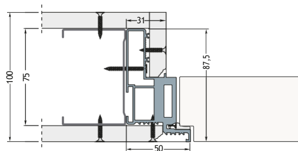
Tokszerkezet egy gipszkarton lappal: Kész fal vastagsága 100 mm
