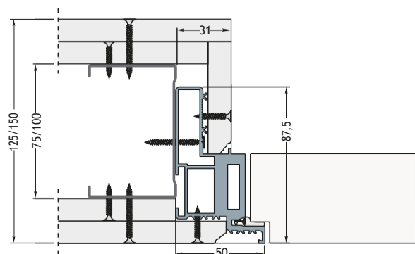
Tokszerkezet két gipszkarton lappal (75 mm-es bordához): Kész fal vastagsága 125 mm
