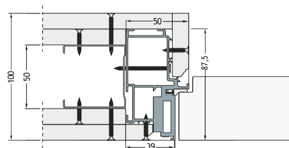
Tokszerkezet két gipszkarton lappal (50 mm-es bordához): Kész fal vastagsága 100 mm
