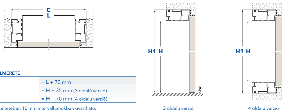
3 oldalú verzió
