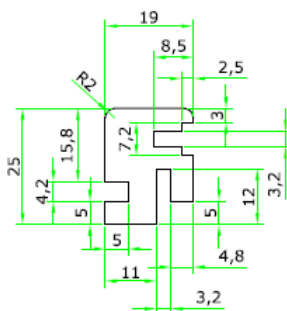
(B) Függőleges tokprofil
