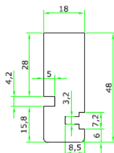
(A) Vízszintes felső tokprofil
