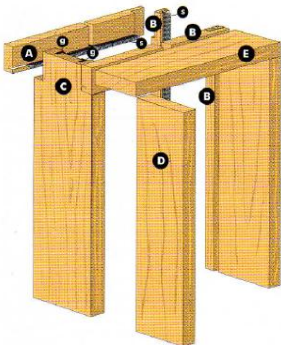
(C) (D) Függőleges belső tokborítás
