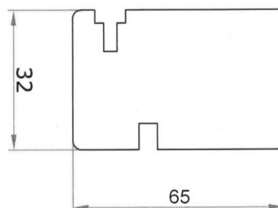
A Vízszintes felső tokprofil
