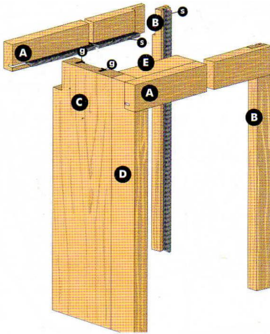
(C) (D) Fügőleges belső tokborítás
