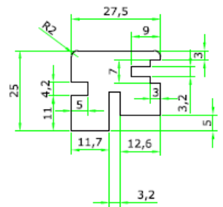
(B) Fügőleges tokprofil
