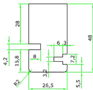
(A) Vízszintes felső tokprofil
