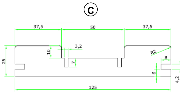
(C) (D) Fügőleges belső tokborítás
